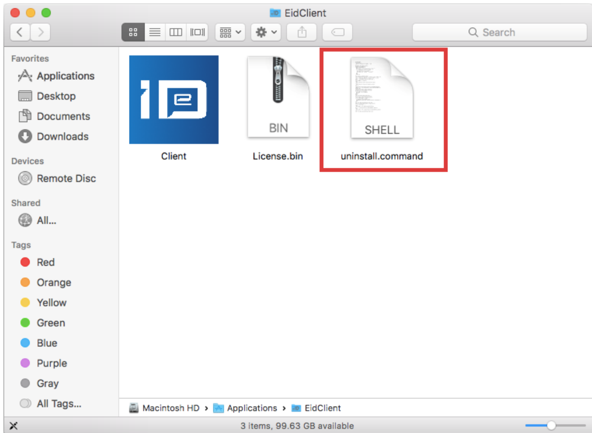
Slika 2.1 Uninstall skripta
