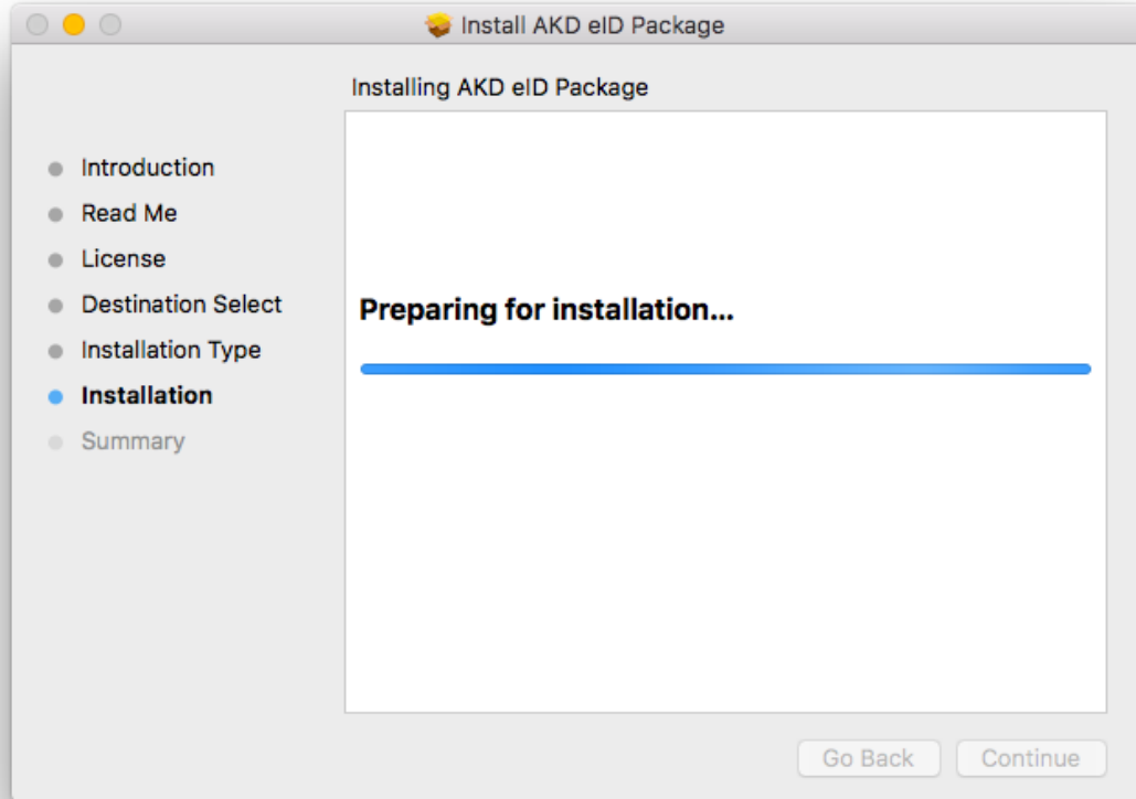
Slika 1.5 Dovršetak instalacije
