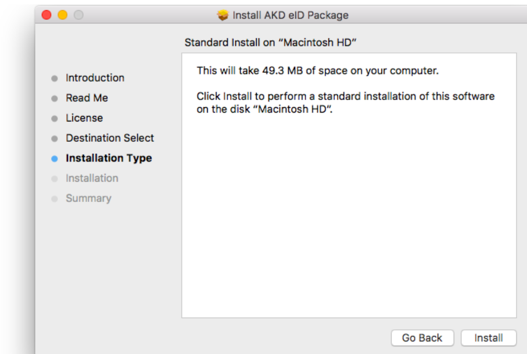
Slika 1.4 Dovršetak instalacije
